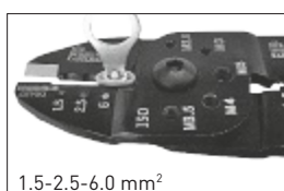
Crimping pliers for insulated terminals Alicate para engastar terminales no aislados Crava terminais isolados
