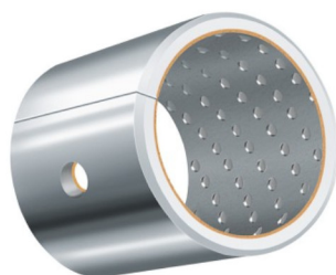
Casquilhos de fricção de material composto de metal-polímero
